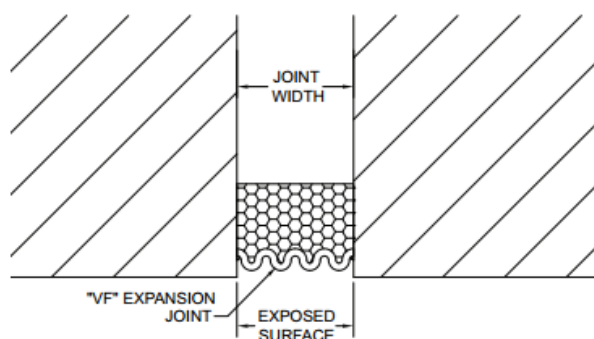
VF (Typ.)
