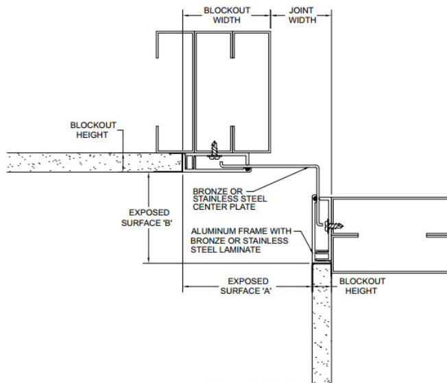
AFWC-S/B (TYP.)
