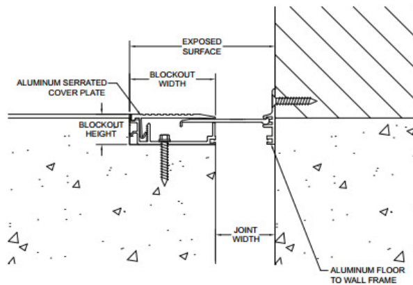
ALSW (TYP.)
