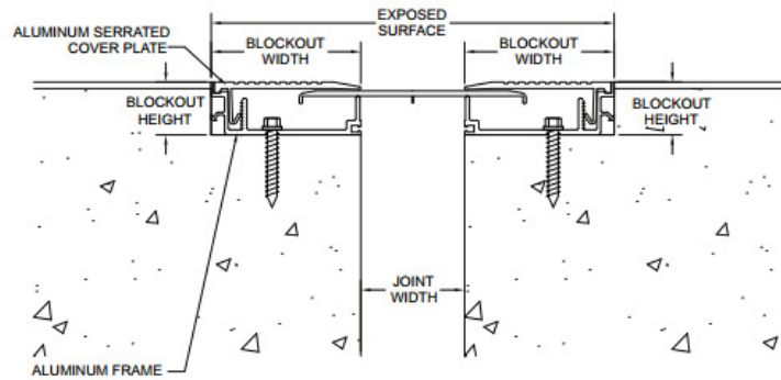
ALS (TYP.)
