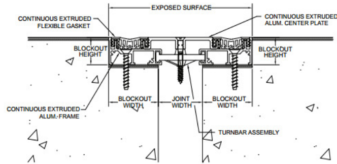
DGTP (TYP.)
