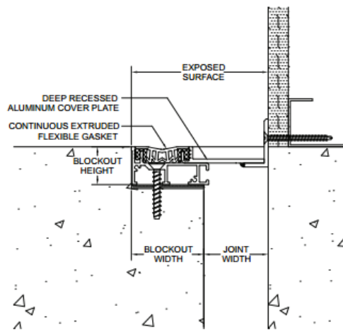
DGTRW-D (TYP.)
