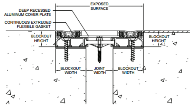
DGTR-D (TYP.)
