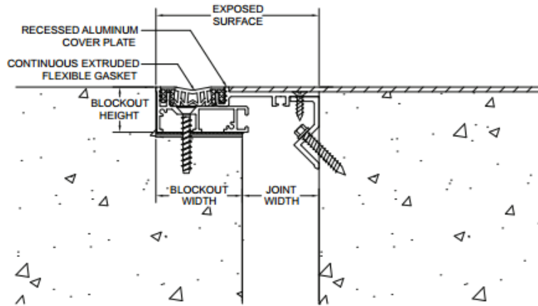
DGTR-M (TYP.)
