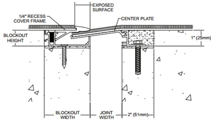
FYW-D (TYP.)
