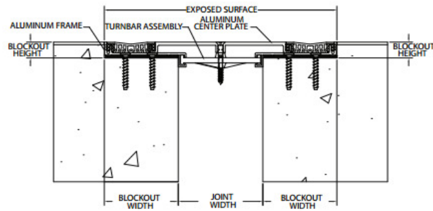
GTP (TYP.)
