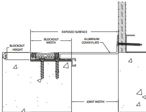
GTPW (TYP.)
