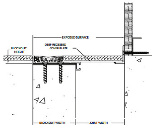
GTRW-D (TYP.)
