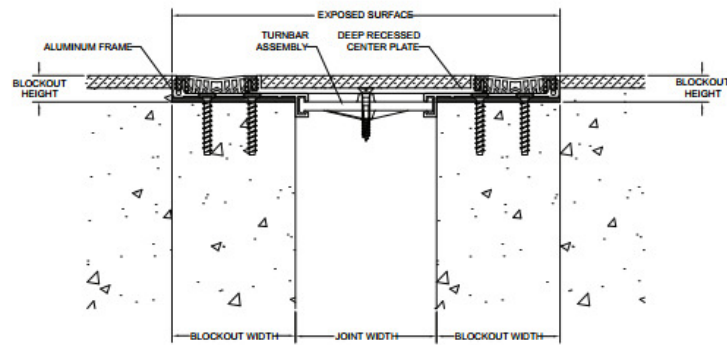
GTR-D (TYP.)
