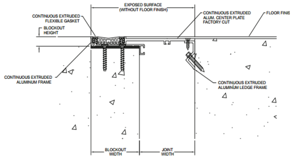
GTR-M (TYP.)
